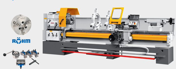
Universal-Drehmaschine mit 3-Achs-Digitalanzeige PREMIUM CU 630 RD - Vario elmag.at/88641
