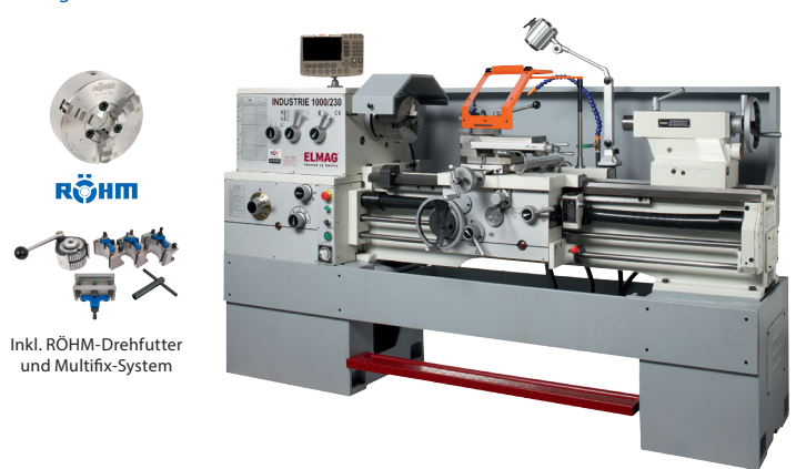
Universal-Drehmaschine INDUSTRIE 1000/230 K elmag.at/88165
